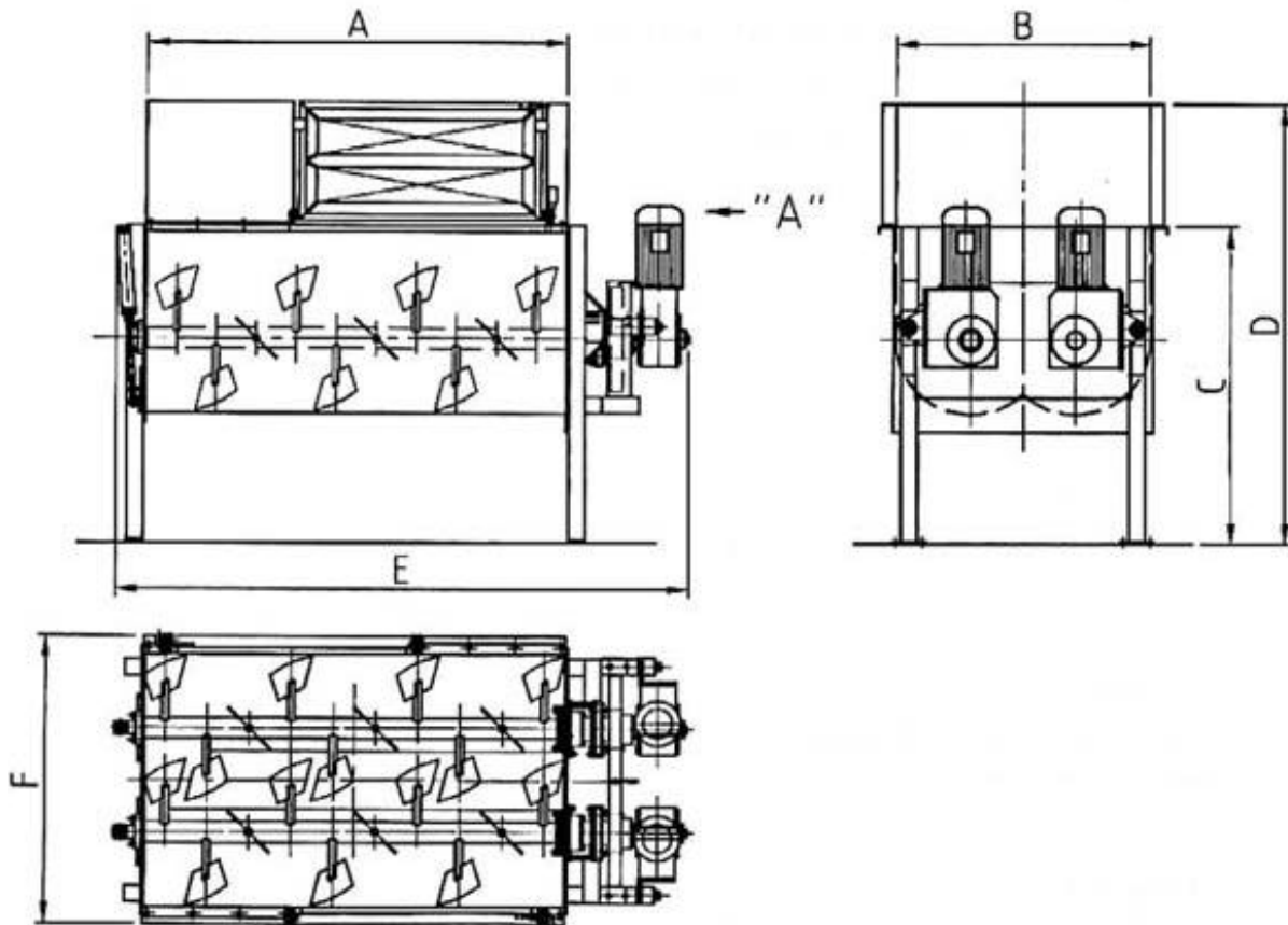
Ansicht „A“
